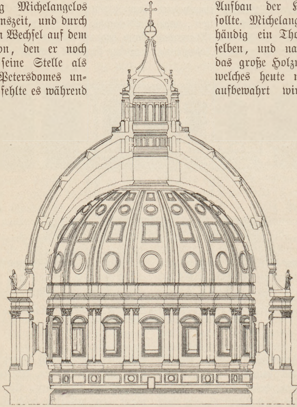
Abb. 92. Durchschnitt von Michelangelos Modell für die Kuppel der St. Peterkirche in Rom.
