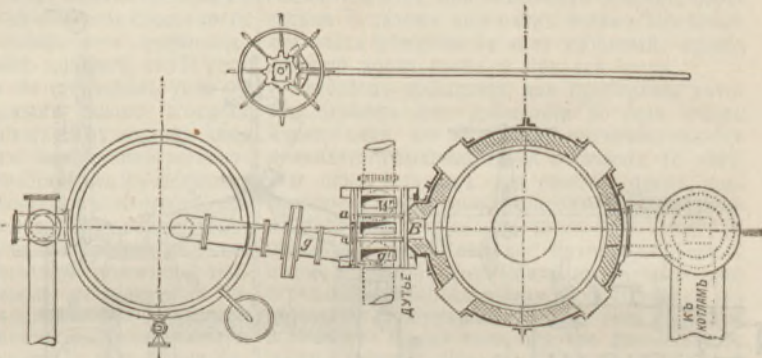
Фиг. 2. Поперечный разрѣвъ прибора, изображеннаго на фиг. 1.
