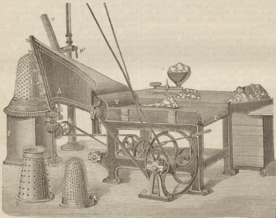
Машина для производства войлочныхъ шляпныхъ колопазовъ.
