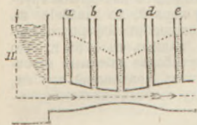
Фиг. 3. Опытъ Фроуда.
