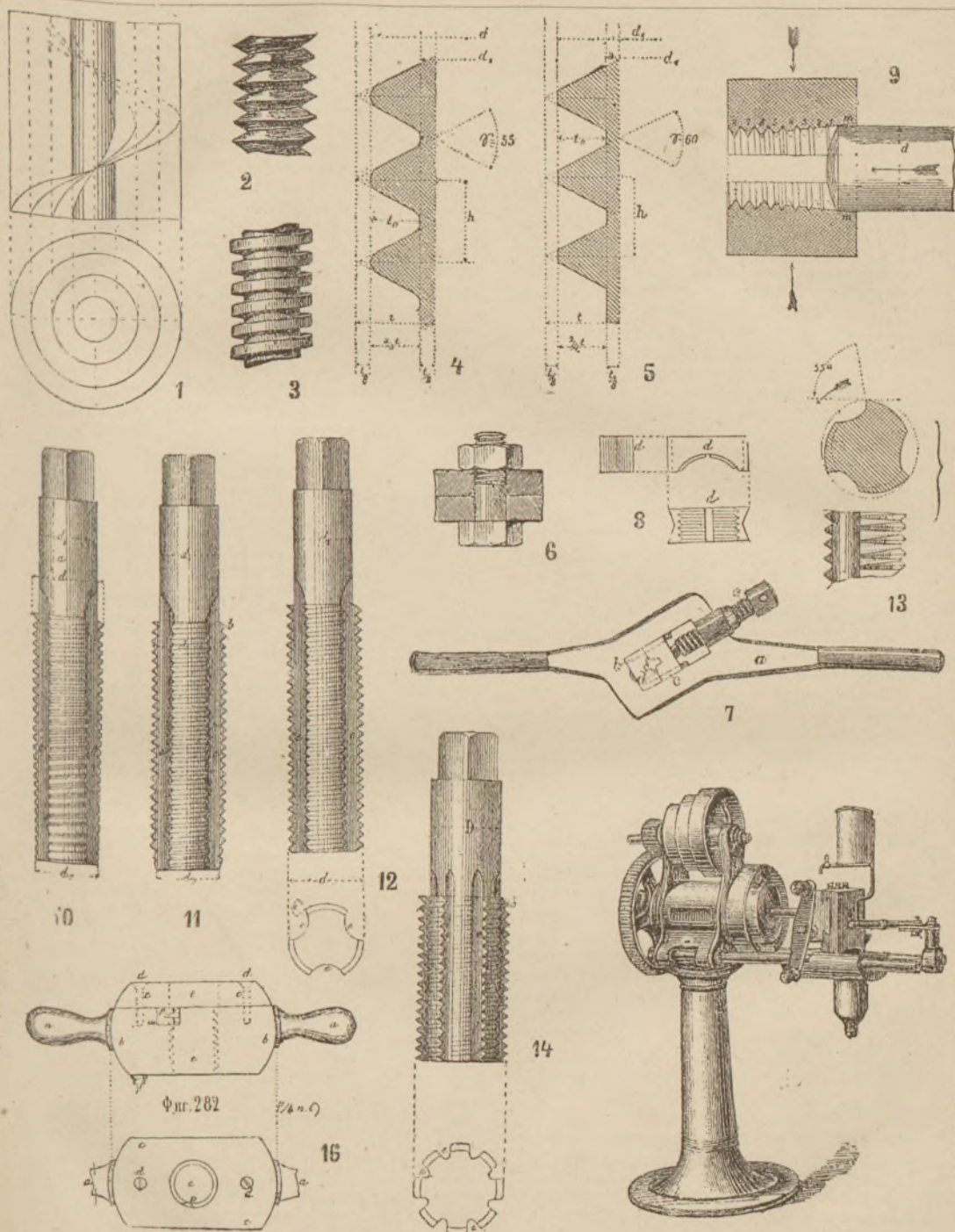
1) Винтовая линия. Нарѣзки: 2) треугольная, 3) квадратная. 4) Витворта. 5) Селзерса. 6) Болтъ. 7) Клупка. 8) Плани. 9) Дѣйствіе плашек Селзерса. 10 и 11) Матчии коническіе. 12) Цилиндрической. 13) Селзерса. 14) Нормальный. 15) Болторѣзная машина. 16. Винтельна.
