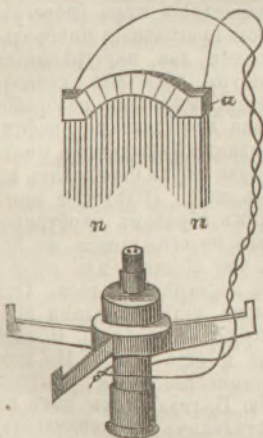
фиг. 3. Гребень Фанельма, а — желобъ изъ жести, наполненный глиной, въ который упрявляются иголки п.
