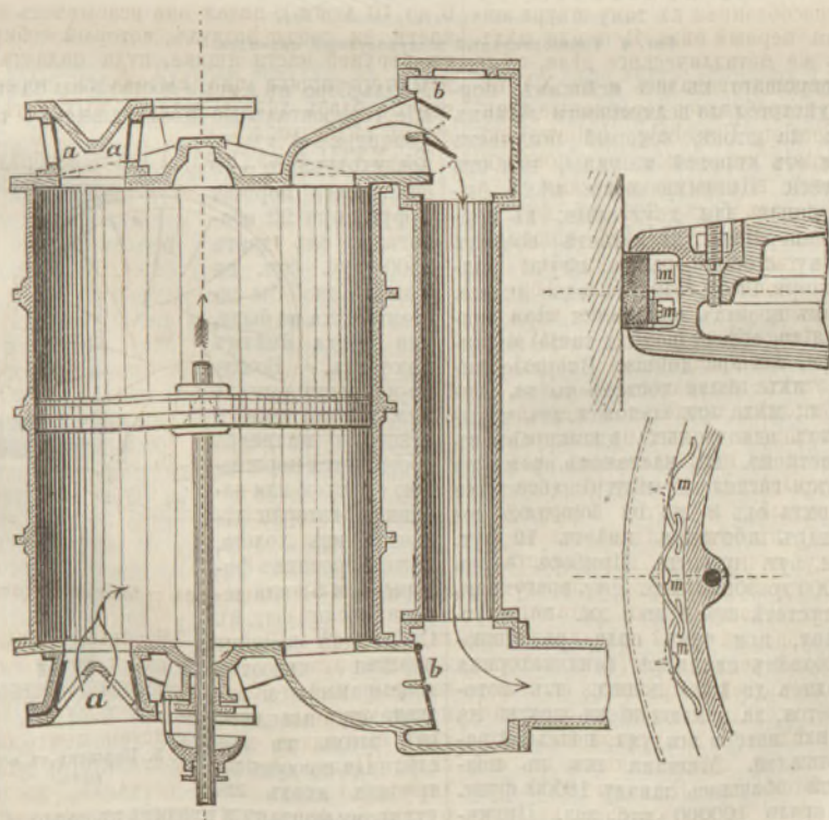
Фиг. 3. Вертикальный воздуходувный цилиндръ (справа, сбоку приспособленіе деревянныхъ «косынокъ» для плотности прилеганія поршня).
