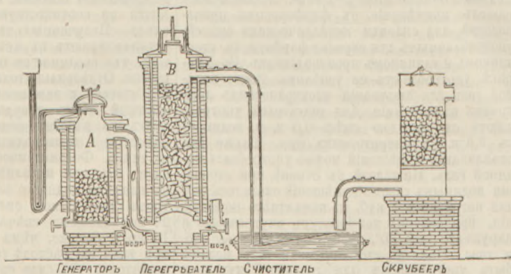
Фиг. 4. Приборъ Лоу для добычянія карбурованнаго водяного газа
