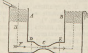
Фиг. 4. Изъ опытовъ Фроуда.
