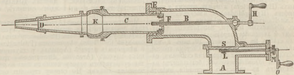
Фиг. 7. Воздухоносный фонтанъ и сопло.
