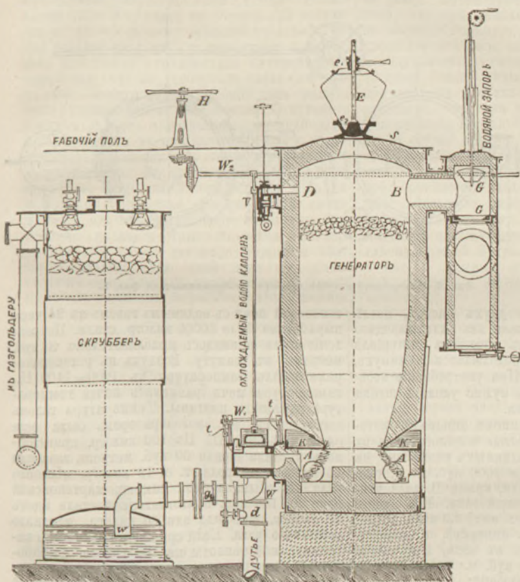
Фиг. 1. Приборъ, примѣняемый въ Эссенѣ для полученія водянаго газа.
