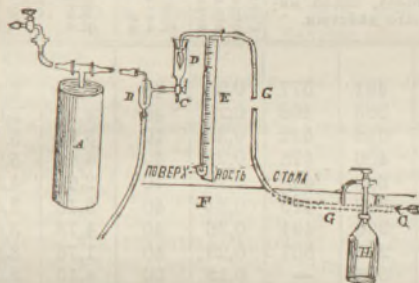
Фиг. 10. Лабораторное приспособленіе къ В.-В. насосамъ В, съ манометромъ Е, показывающимъ степень разряженія.
