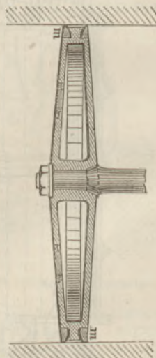
Фиг. 5. Поршень съ воротничкомъ.
