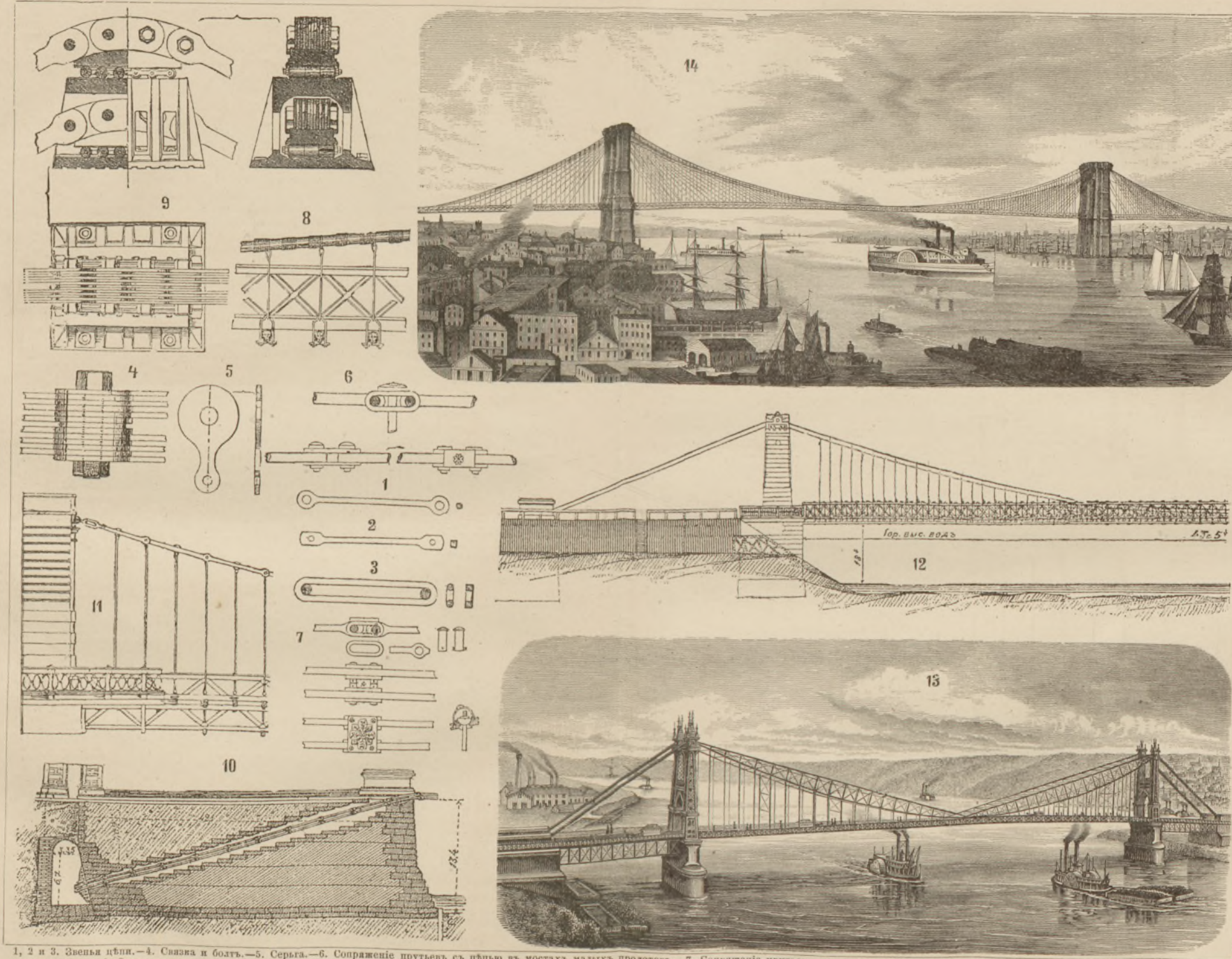
1, 2 и 3. Звенья цѣпи.—4. Связка и болтъ.—5. Серьга.—6. Сопряженіе прутьевъ съ цѣпью въ мостахъ малыхъ пролетовъ.—7. Сопряженіе прутьевъ съ цѣпью въ Маикопскомъ мостѣ въ С.-Петербурѣ.—8. Деталь канатнаго моста.—9. Опорная тележка для цѣпей.—10. Устой.—11. Деталь Николаевскаго цѣпнаго моста чрезъ р. Днѣпръ въ Кіевѣ.—12. Полупродѣлъ цѣпнаго моста чрезъ р. Великую въ Островѣ.—13. Цѣпной мостъ въ Псковѣ.—14. Проволочно-канатный мостъ чрезъ East-River въ Нью-Йоркѣ.
