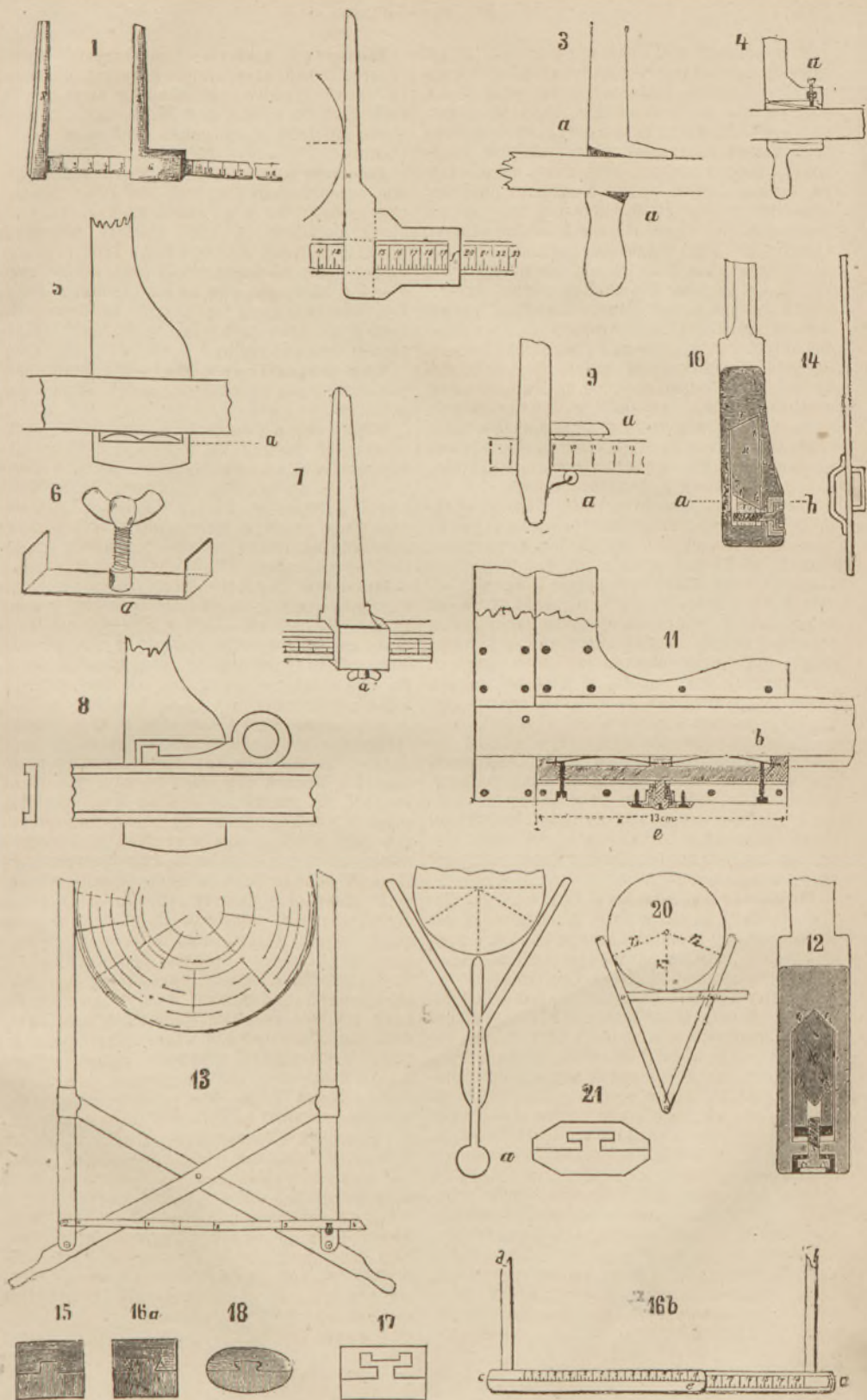
В. 1 и 2. Первоначального устройства; 3. Альденбика; 4. Вёмерле; 5. Тарандская; 6 и 7. Карла Гейера; 8. Смаляная; 9. Шульце; 10. Густава Гейера; 11. Нейге-ера; 12. Эд. Гейера; 13. Литкена; 14. Отена; 15. Пюшеля; 16 а и б Фридриха; 17. Вагнера; 18. Гандлосса; 19. Кольберга; 20. Трезурта и 21. Петровская.
