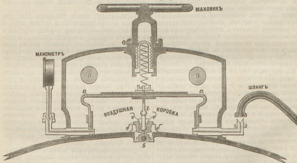
Цилиндръ аккумулятора.
