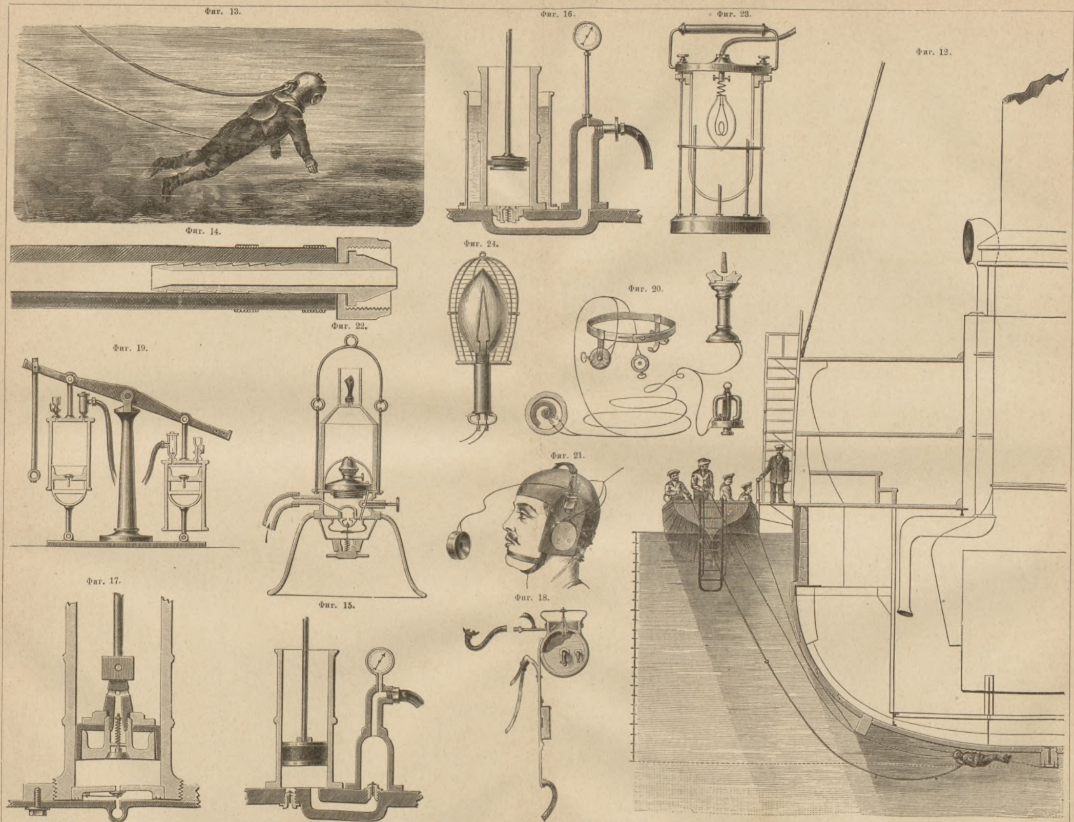
Фиг. 12.—Мидельшпангоут современного Фрегата («Дмитрий Донской») у трапа; вооруженная водолазная шлюпка, а между ними показано положение работающего водолаза; Фиг. 13.—Ходячие водолазы по дну, когда они ныряют; Фиг. 14.—Разрыв воздухопроводной шланга и соединительной медной трубки с гайкою (1/2 нат. велич.); Фиг. 15.—Разрыв Помпы «Гейлесс» (Зибе, Горюнов и К о ); Фиг. 16.—Разрыв Помпы Декейруа с холодильником; Фиг. 17.—Помпа Шрадера; Фиг. 18.—Равец Декейруа; Фиг. 19.—Гидравлическая малая водолазная помпа с 2 качающимися цилиндрами—Декейруа; Фиг. 20.—Телефонные приспособления водолазной школы; Фиг. 21.—Новейшие телефонные аппараты для водолазов; Фиг. 22.—Подводное освещение Декейруа; Фиг. 23.—Подводный электрич. фонарь лейтенанта Твриттинова; Фиг. 24.—Подводное освещение по систем водолазного офицера лейтенанта Колбасева.
