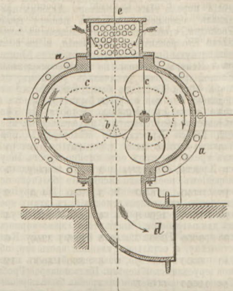
Фиг. 1. Вентиляторъ Рута.
