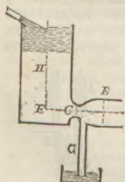
Фиг. 5. Подъемъ воды отъ уменьшенія давленія въ C .
