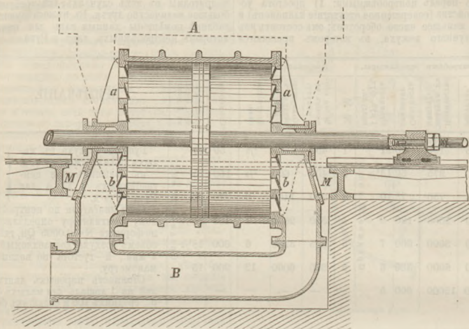
Фиг. 4. Горизонтальный воздуховый цилиндръ.
