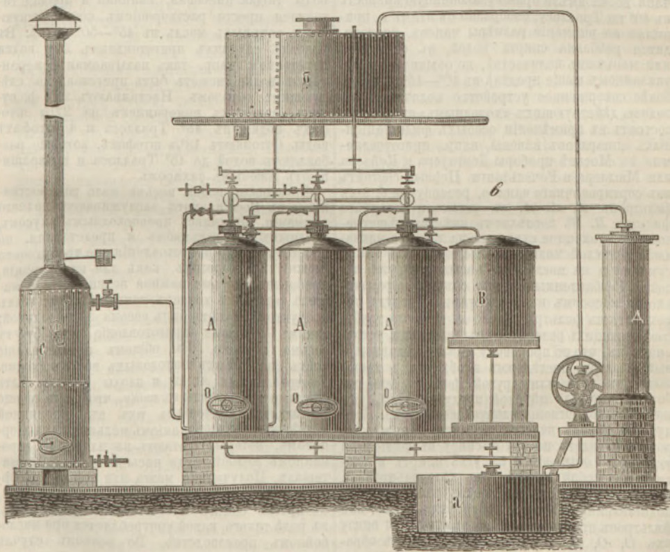
Приборъ для «холоднаго» очищенія водки отъ вредныхъ частей сивушнаго масла, при помощи процеживанія черезъ уголь.
