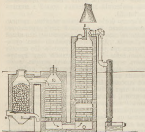
ГЕНЕРАТОРЪ КАРБУРАТОРЪ ПЕРЕГРѢВАТЕЛЬ НЕПРѢВѢТѢЛЬ МАСЛА Фиг. 5. Усовершенствованное устройство прибора Лоу.
