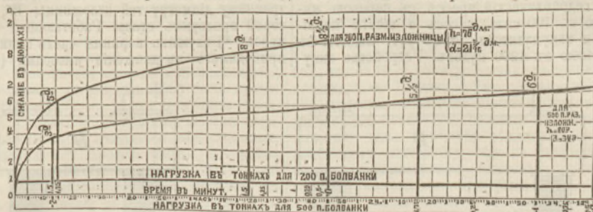
Фиг. 3. Диаграмма, выражающая сжатие, в дюймах, остывающей стальной болванки при разных давлении, производимых прессом Витворта.
