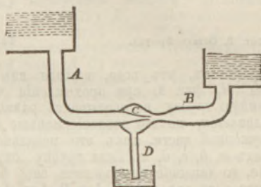
Фиг. 1. Схема водоструйного насоса Томсона.
