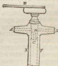
Фиг. 11. Сообщающій кранъ.
