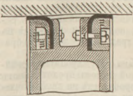
Фиг. 6. Воротникъ поршня.
