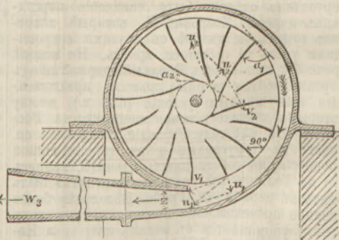
Фиг. 2. Центробѣжный вентиляторъ съ быстрымъ вращеніемъ.
