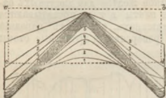
Фиг. 6. Послѣдовательное измѣненіе формъ желѣзной (и стальной) полосы при полученіи углового желѣза.
