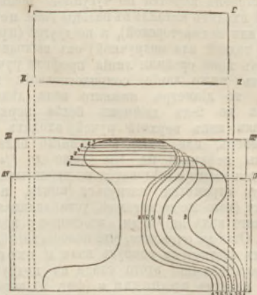
Фиг. 5. Послѣдовательное измѣненіе пакета при прокатѣ рельсоваго желѣза (и стали).
