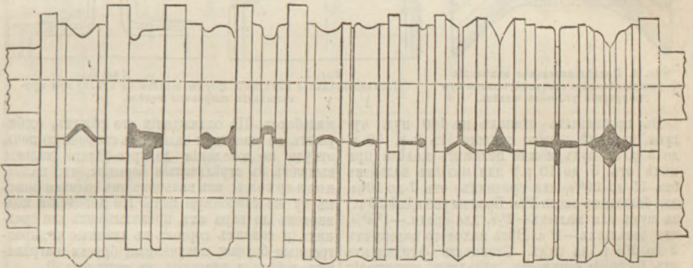
Фиг. 3. Отдѣльные ручки прокатныхъ вальцовъ для получения различныхъ сортовъ фасоннаго желѣза (и стали).
