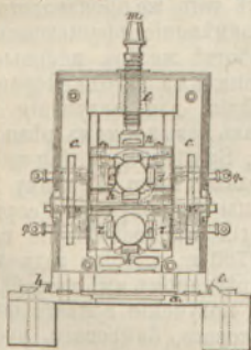
Фиг. 2. Прокатный станъ, какъ на фиг. 1. Поперечный разрѣзъ.
