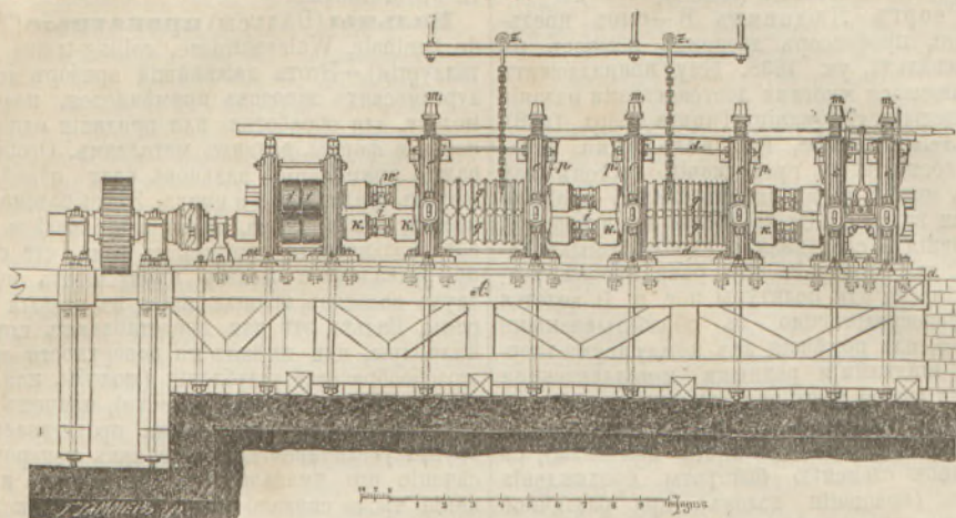
Фиг. 1. Прокатный станъ для получения сортового желѣза (и стали). Общій продольный видъ.
