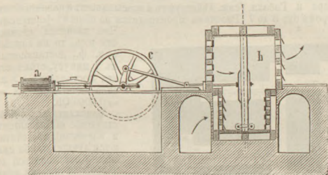
Рудничный поршневой вентиляторъ системы Никсона. Поршень b движется въ моментъ изображенія на рис. съ лѣва направо, а потому высасываніе идетъ изъ лѣваго устья, какъ видно по положенію клапановъ.
