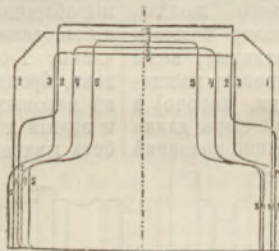
Фиг. 7. Послѣдовательное измѣненіе формы желѣза (и стали) при прокатываніи тавроваго желѣза.
