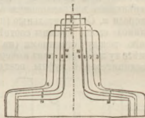
Фиг. 7. Послѣдовательное измѣненіе формы желѣза (и стали) при прокатываніи тавроваго желѣза.
