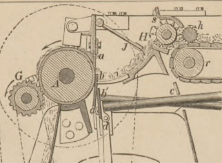
2. Ножевая зерноочистительная машина (ножевый джигъ).
