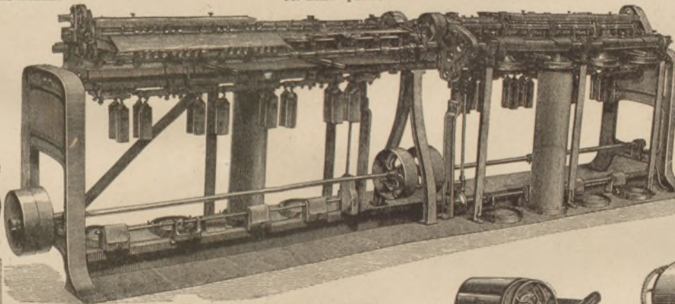
12. Ленточная вытяжная машина.
