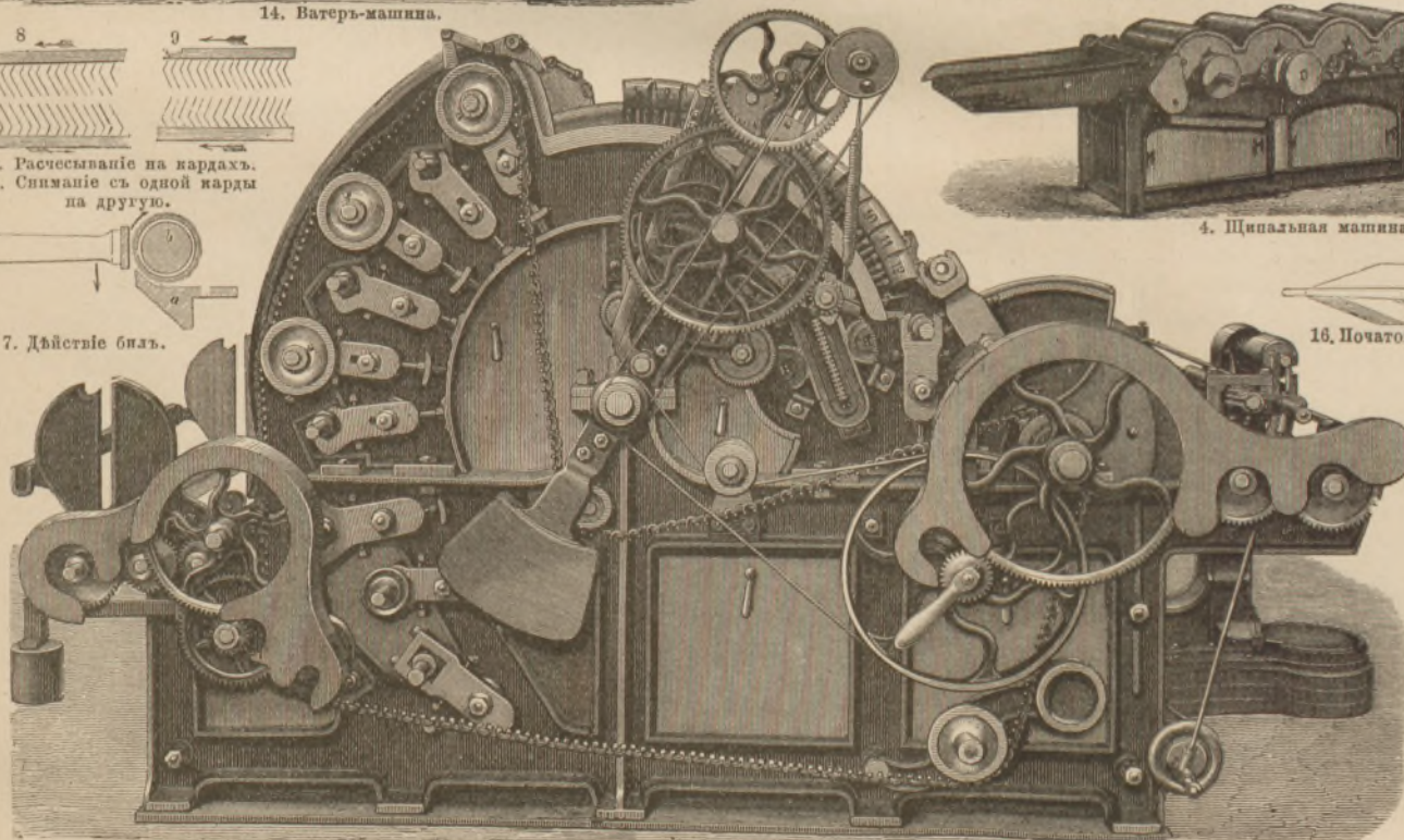
10. Смѣшанная кардъ-маш. (мьясть).
