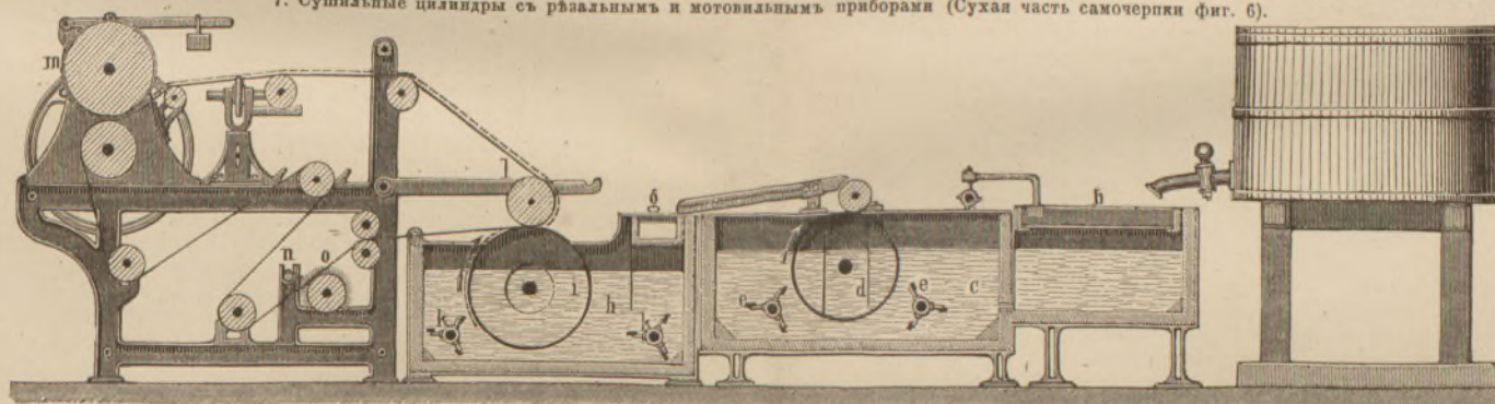
9. Цилиндрическая папковая машина.
