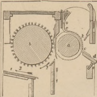
1. Пиляная зерноочистительная машина (пиляный джигъ).
