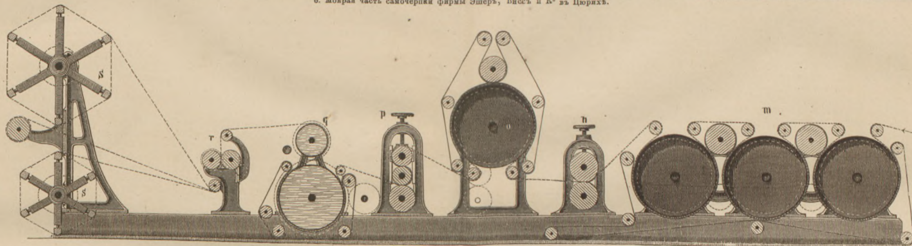
7. Сушильные цилиндры съ рѣзальнымъ и готовильнымъ приборами (Сухая часть самочерпни фиг. 6).
