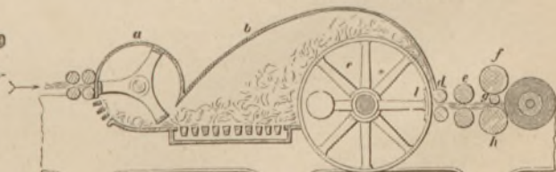
5. Трепальная машина прежней конструкціи.
