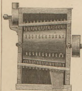
2. Волкъ-машина (пыле-отбиватель).
