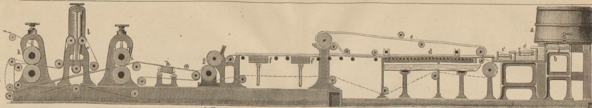
6. Мокрая часть самочерпни фирмы Эшеръ, Виссэ и К° въ Цюрихѣ.
