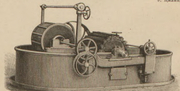
3. Роль съ промывнымъ барабаномъ.
