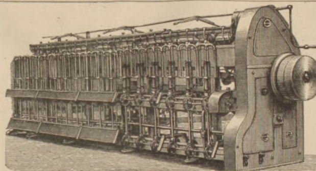
13. Банкаброшъ.
