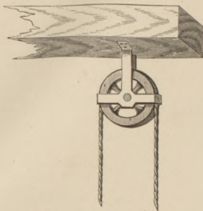
3. Блокъ-Полнспасть.
