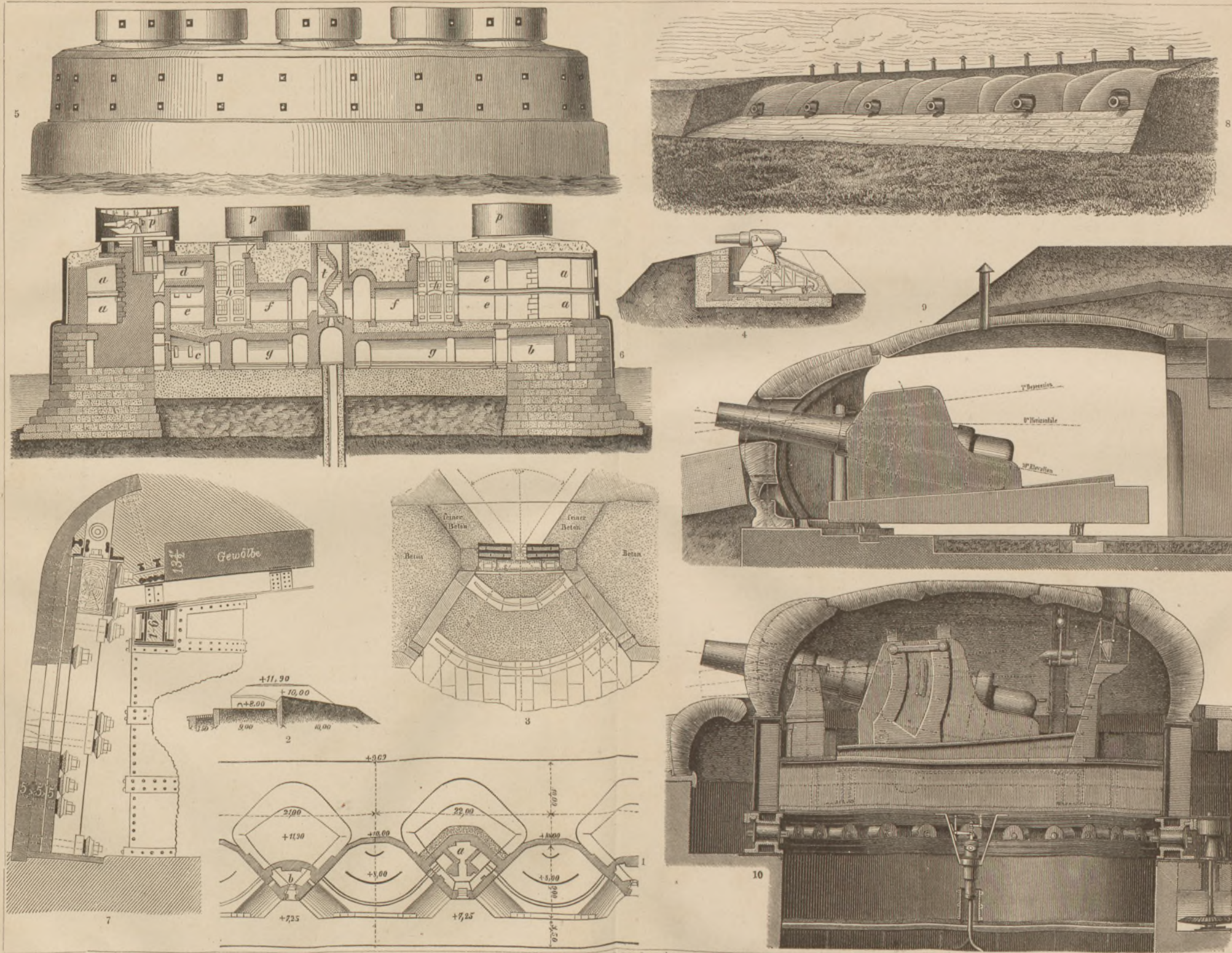
1) Германскій береговой фортъ: линия орудейныхъ помѣщеній, въ планѣ. 2) Профиль середины одного орудейнаго помѣщенія, какъ изображенныхъ на фиг. 1. 3) Англійскій нормальный береговой фортъ: амбразура съ броневымъ щитомъ. 4) Орудіе на лафетъ Монкрифа, готовое къ дѣйствію. 5) Внѣшній видъ форта Спитхедъ (въ Портсмутѣ). 6) Фортъ Спитхедъ (Портсмутъ) въ разрѣзѣ. 7) Фортъ Брекуатеръ (Плимутъ): броневая одежда въ разрѣзѣ. 8) Внѣшній видъ броненосной батареи для шести пушекъ калибра 24 см. (Gruson Patent). 9) Броненосная батарея для шести пушекъ калибра 24 см. (Gruson Patent), въ разрѣзѣ. 10) Броненосная башня для двухъ орудій, калибра 28 см. (Gruson Patent), въ разрѣзѣ.
