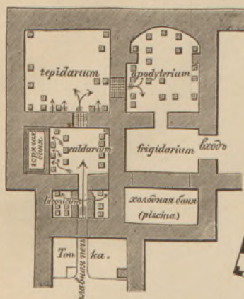
Планъ римскихъ бань въ Кар- вентъ (Aptaria).
