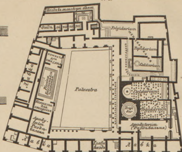
Планъ термъ въ Помпеяхъ.
