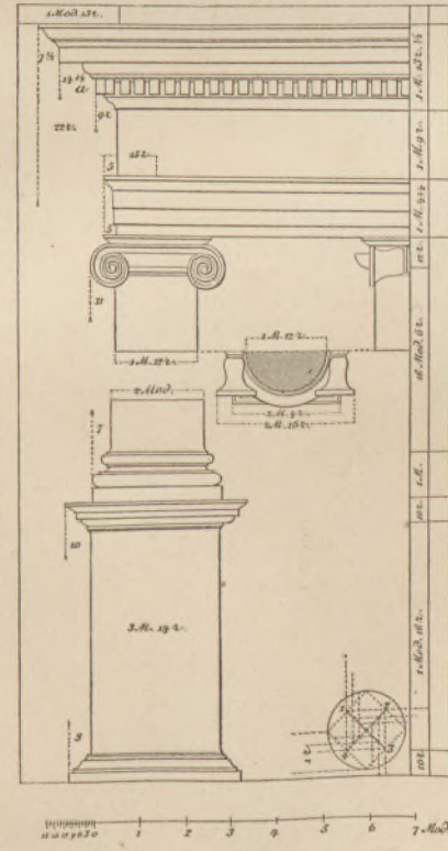
Черт. 14-й. Ионическій орденъ.
