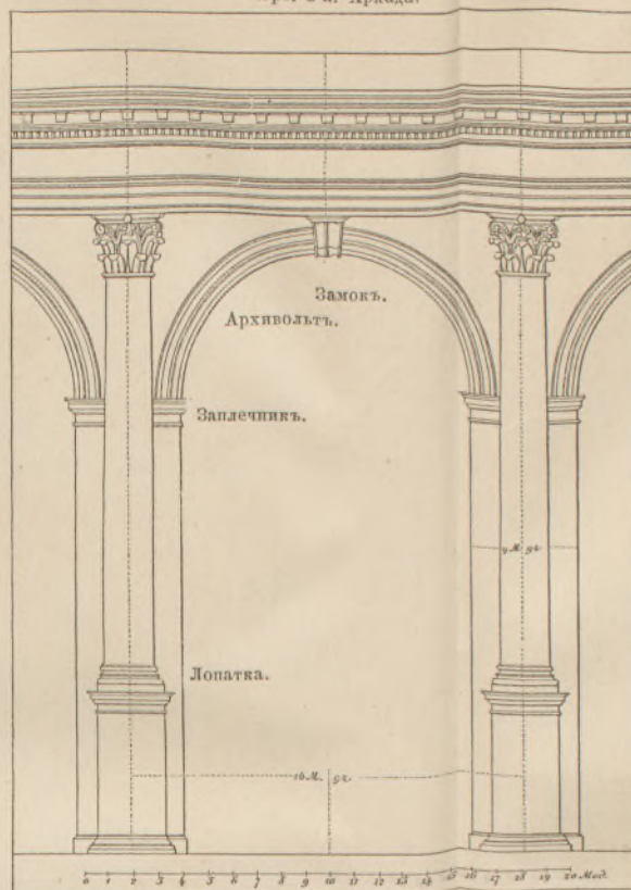
Черт. 12-й. Сложн. капит.
