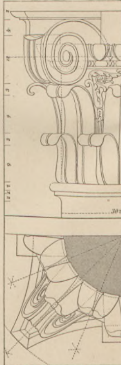
Черт. 12-й. Сложн. капит.
