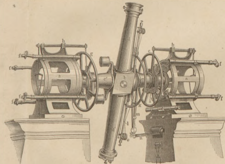
Фиг. 1. Меридианный кругъ Страсбургской Обсерватории. Построенъ бр. Репсольдъ въ Гамбургъ, объективъ Мерца въ Мюнхенъ, отверстие объектива 16, сант., фокусное расстояние 1,2 метровъ.
