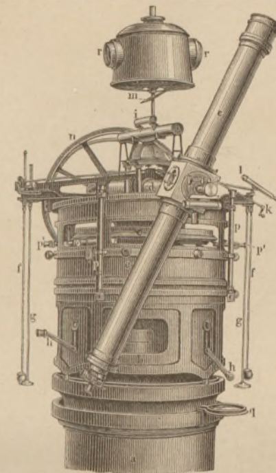
Фиг. 3. Альтазимут Страсбургской Обсерватории. Объектив Мерца в Мюнхен, механическая часть бр. Репсольд в Гамбург. Диаметр цилиндра 84 сант., отверстие объектива 13,2 сант., фокусное расстояние 1,5 метра.
