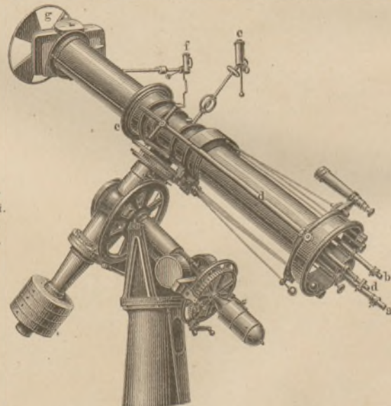
Фиг. 4. Гониометръ Обсерватори въ Нью-Гавенъ (Съв. Ам.). Построенъ бр. Репсольдъ въ Гамбургъ.
