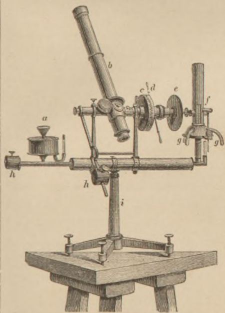
Фотометръ Цейснера (Къ ст. „Астрофотометрія“).
