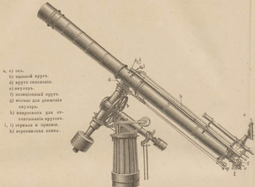
Фиг. 2. Большой рефрактор Страсбургской Обсерватории. Объектив Мерца в Мюнхен, механическая часть бр. Репсольд в Гамбург. Диаметр объектива 48,7 сант., фокусное расстояние 7 метров.
