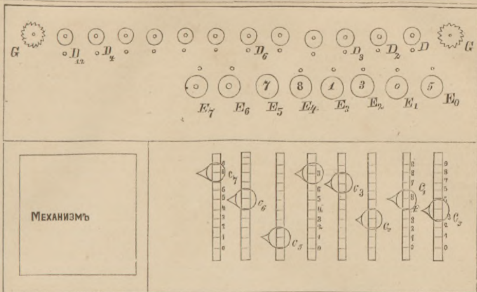
Схематическій черт. Арифмометра Томаса.
